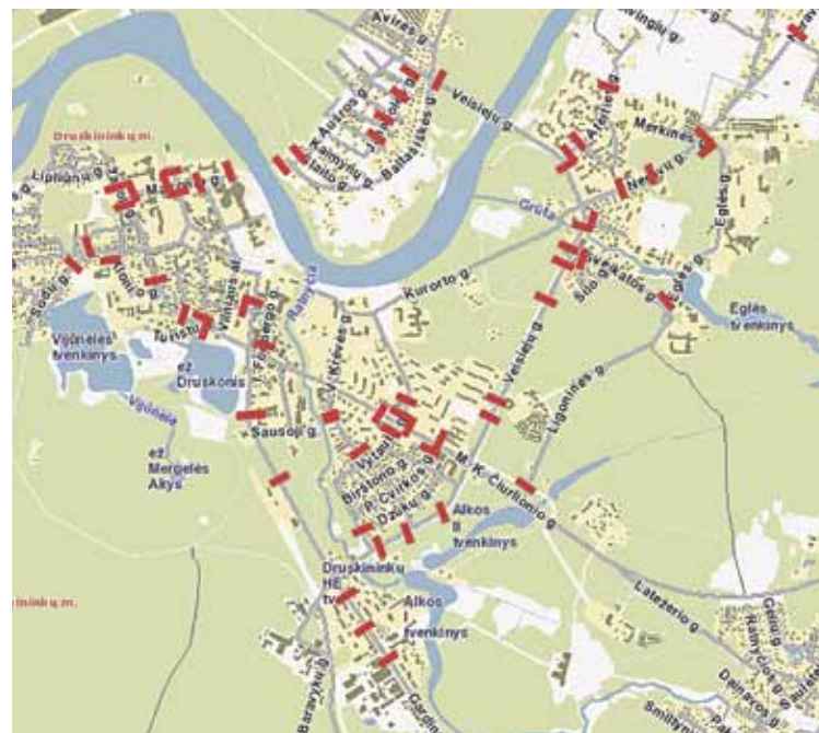
Kryptinio pėsčiųjų perėjų apšvietimo išdėstymo schema Druskininkuose.
