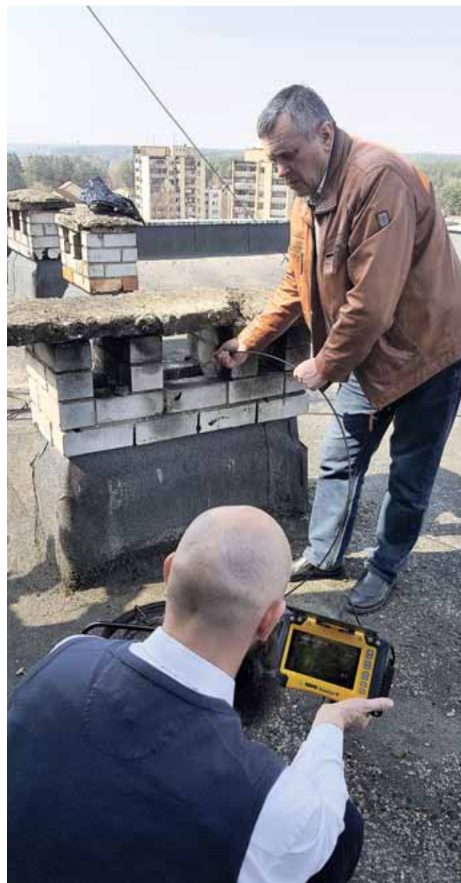
Nustačius vamzdynų defektus, informacija apie juos įrašoma į bendrovės duomenų bazę/Laimos Rekevičienės nuotrauka
